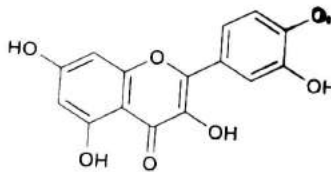
Kuersetin
