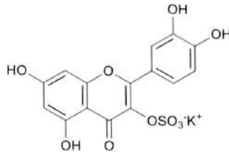
Kuersetin-3-kalium bisulfat
