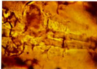
4. Makrosklereida
