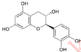
(+) Katekin
