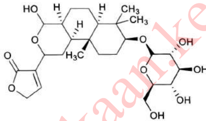
Kurkumangosida
