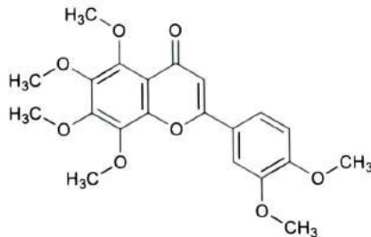
Nobiletin
