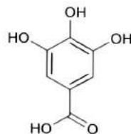
Asam galat
