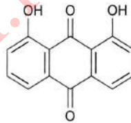
1,8-dihidroksiantrakuinon
