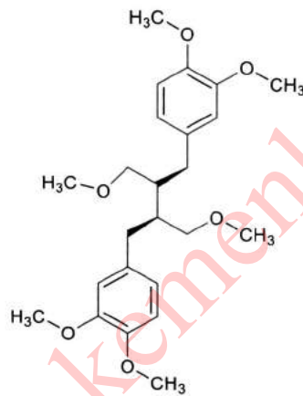
Filantin
