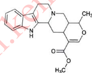
Tetrahidroalstonin
