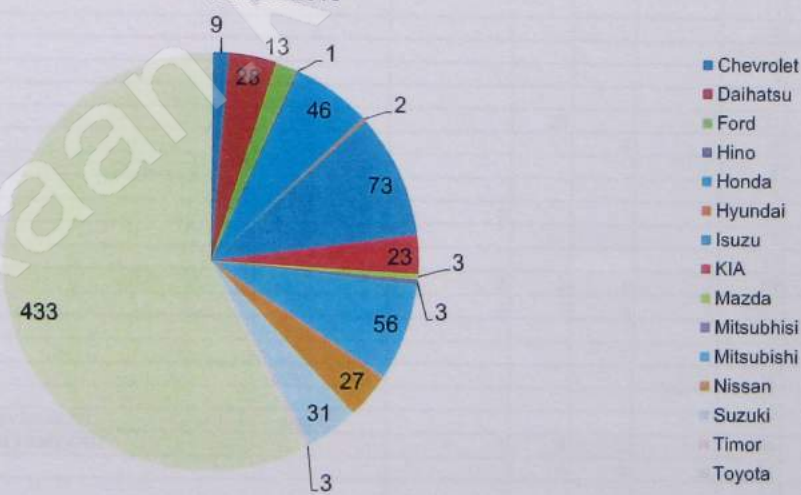
DIAGRAM PERBANDINGAN JUMLAH AADB BERDASARKAN MERK TAHUN 2015
