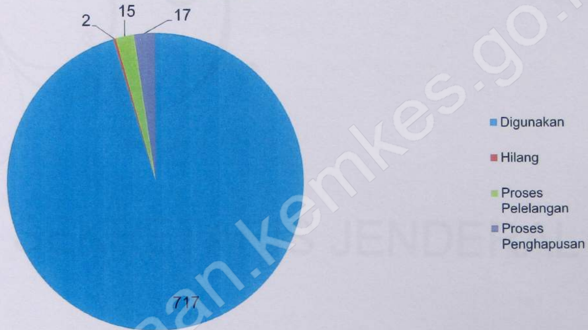
DIAGRAM PERBANDINGAN AADB BERDASARKAN STATUS PENGGUNAAN TAHUN 2015
