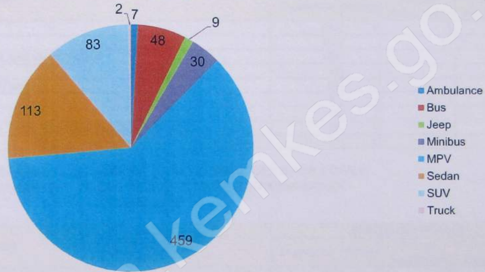
DIAGRAM PERBANDINGAN AADB BERDASARKAN JENIS KENDARAAN TAHUN 2015
