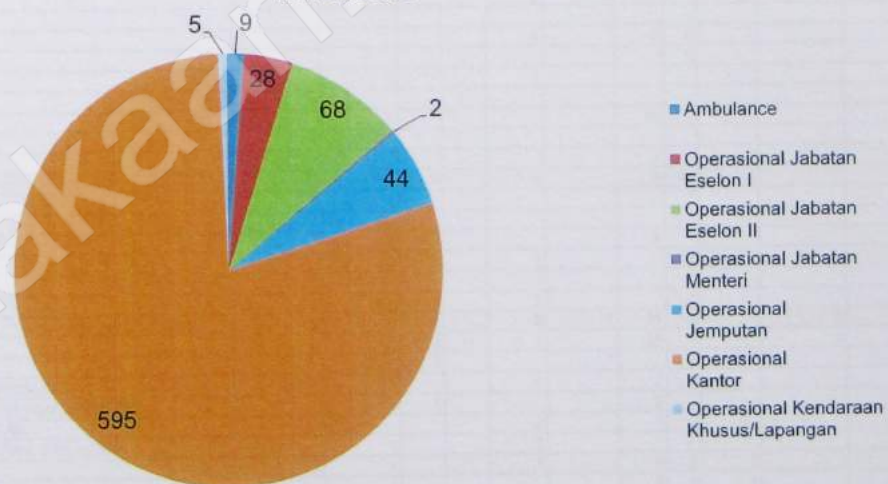
DIAGRAM PERBANDINGAN AADB BERDASARKAN PERUNTUKAN TAHUN 2015
